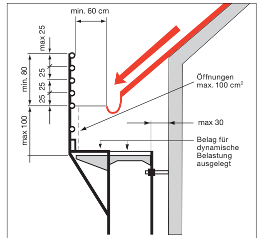
5 Dachdeckerschutzwand für Dächer mit Neigung von 25° und mehr
