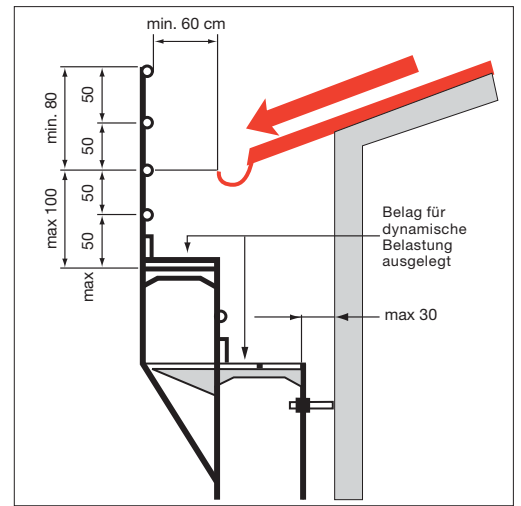
4 Seitenschutz für Dächer mit Neigung bis 25°
